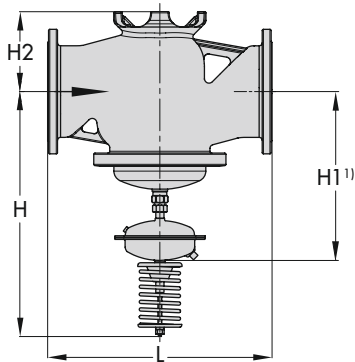
Ventil Typ 2422 membranlastet mit Antrieb Typ 2424
