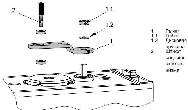
Рис. 5-4: Монтаж рычага и следящего штифта
