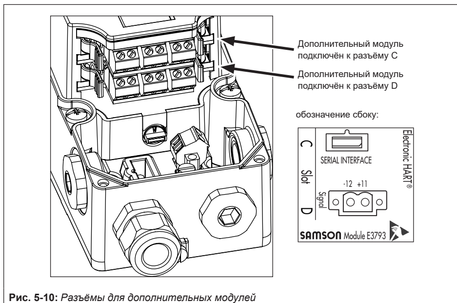
Рис. 5-10: Разъёмы для дополнительных модулей
