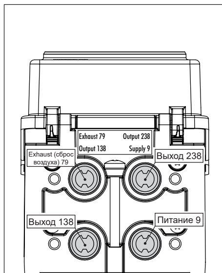
Рис. 5-31: Пневматические выходы
