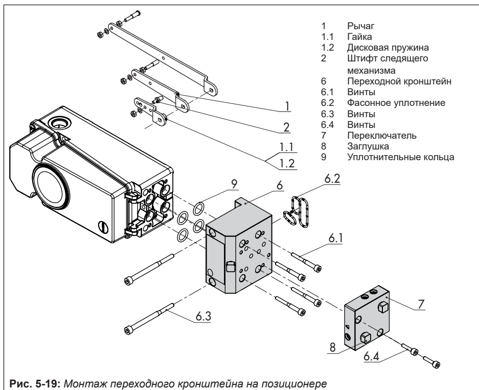
Рис. 5-19: Монтаж переходного кронштейна на позиционере
