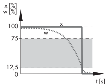
Рис. 3-2: Дискретный анализ заданного значения
